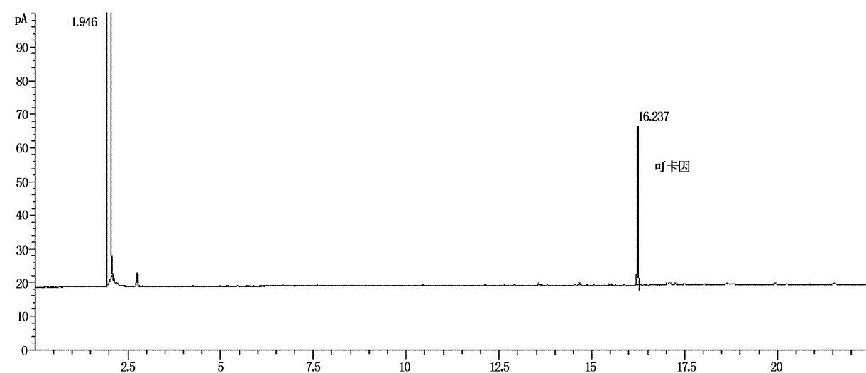
图 B.1 可卡因气相色谱图
