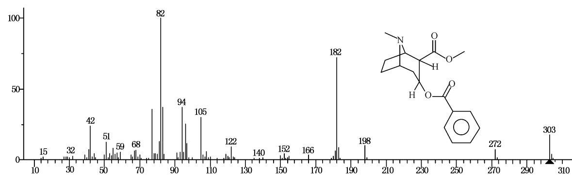
图 B.1 可卡因气相色谱图
